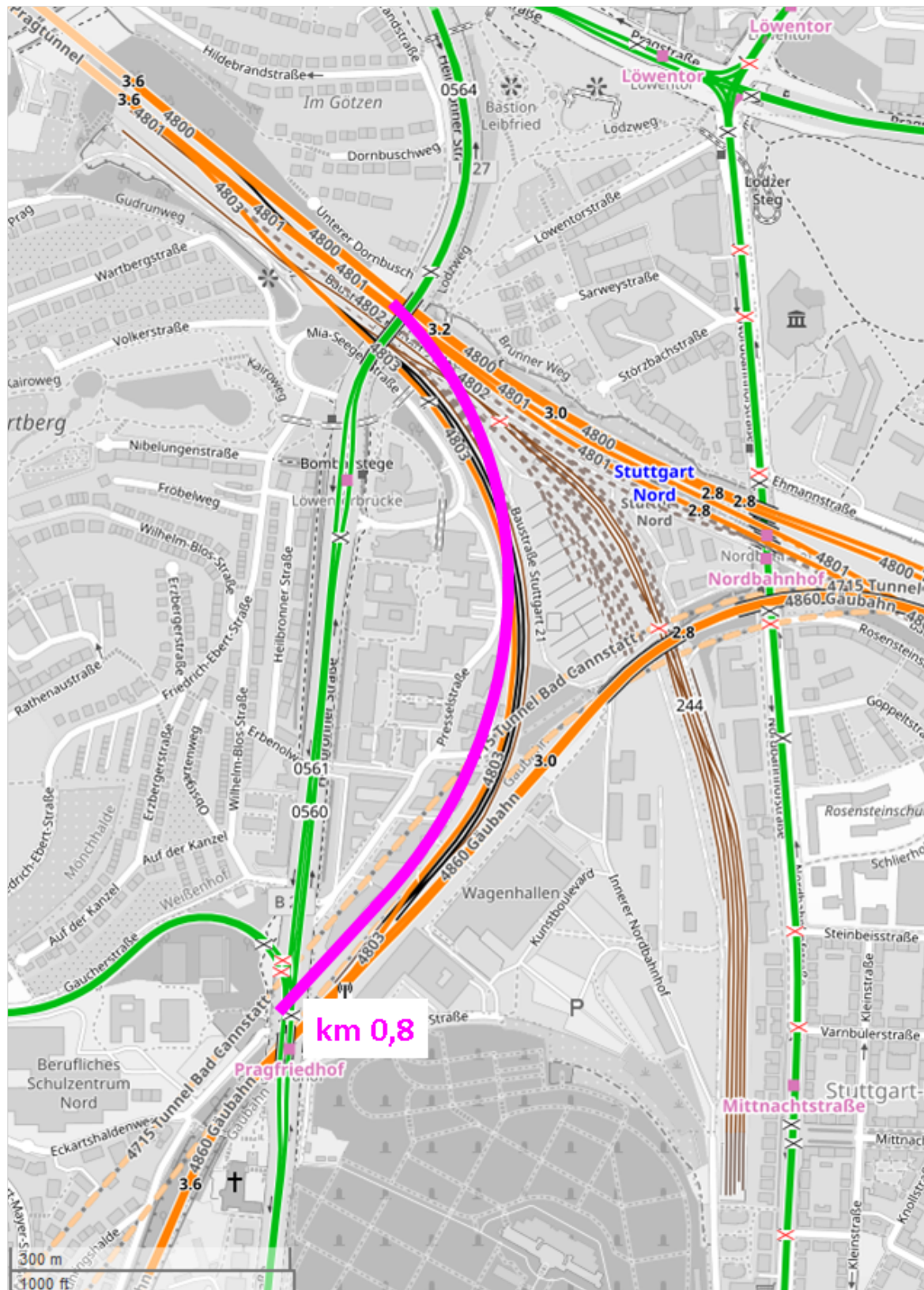
Abbildung 3: Zusatztunnels für Stuttgart 21 Verbindung Feuerbach–Zulauf-tunnels Cannstatt („P-Option“)
