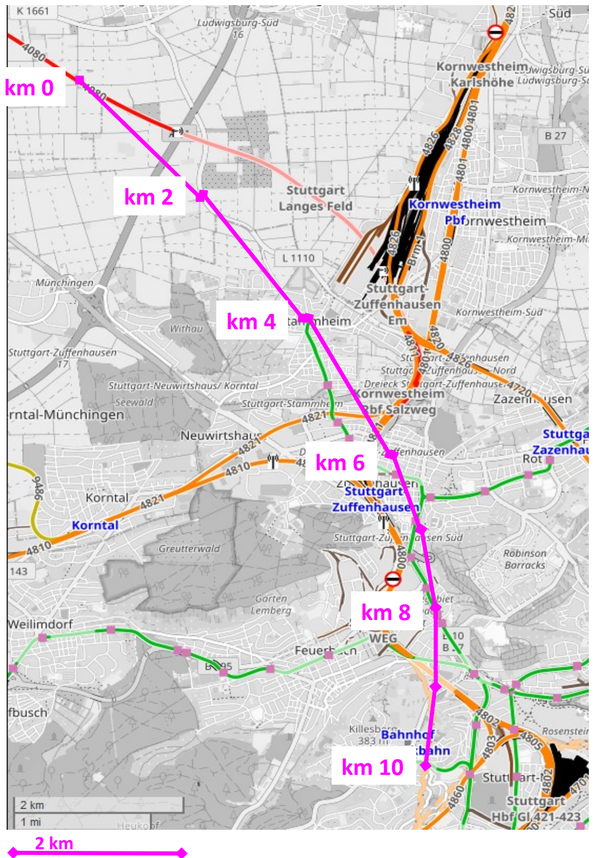
Abbildung 1: Zusatztunnel für Stuttgart 21 Nordzulauftunnel über ca. 10 Kilometer
