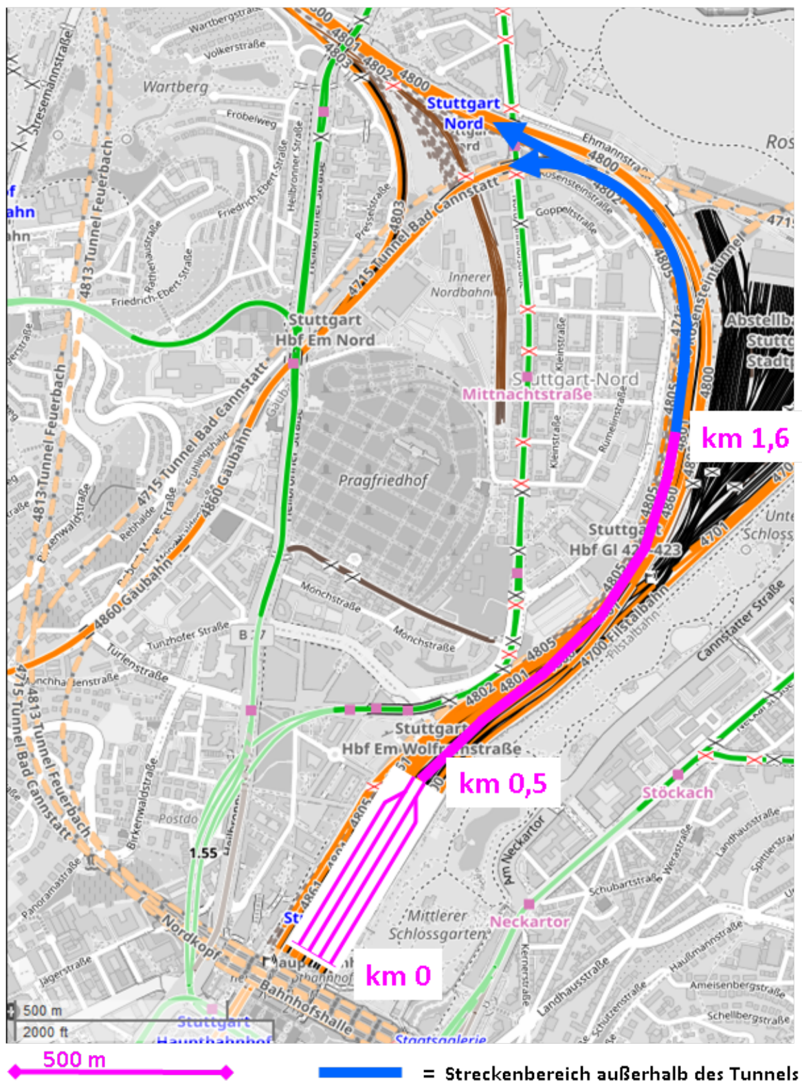
Abbildung 4: Zusatztunnels für Stuttgart 21 Gäubahnzuführung mit Ergänzungs-Kopfbahnhof
